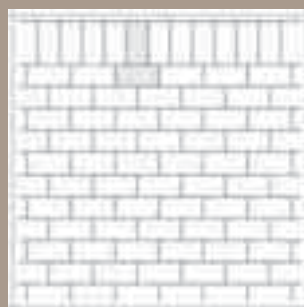
Löpförband i halvformat med rullskift.
