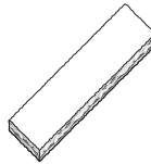
Madoc Mur Toppstén 475x125x40 mm 6 kg/st, 2,1 st/lpm Färger: 39, 40, 44
