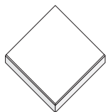
500 Helplatta 500x500x70 mm 160 kg/m 2 , 4 st/m 2 Färger: 10, 12
