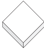
350 Helplatta Ofasad 60 mm 350x350x60 mm 138 kg/m 2 , 8 st/m 2 Färger: 12
