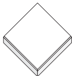
350 Helplatta 60 mm 350x350x60 mm 138 kg/m 2 , 8 st/m 2 Färger: 10, 12, 20
