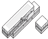
Madoc Mur Helsten 580x100x140 mm 16,5 kg/st, 15,2 st/m 2 Byggglängd 470 mm. Färger: 39, 40, 44
