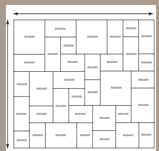
Bradstone Europack förslag, 2,7 x 2,25 m.
