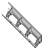
Spikbart kantstöd 1000x80x45 mm En sats innehåller 4 st kantstöd och 12 st stålspik.
