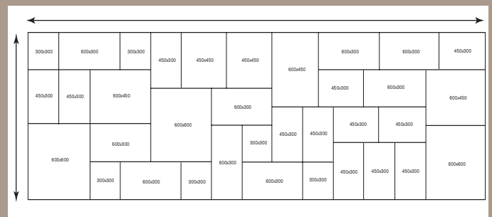
Bradstone Europack förslag, 4,5 x 1,35 m.
