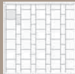
Löpförband med hel- och 1/2-format.
