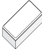
Blocksten Hel 700x350x150 mm 84 kg/st, 9,5 st/m 2 Färger: 12
